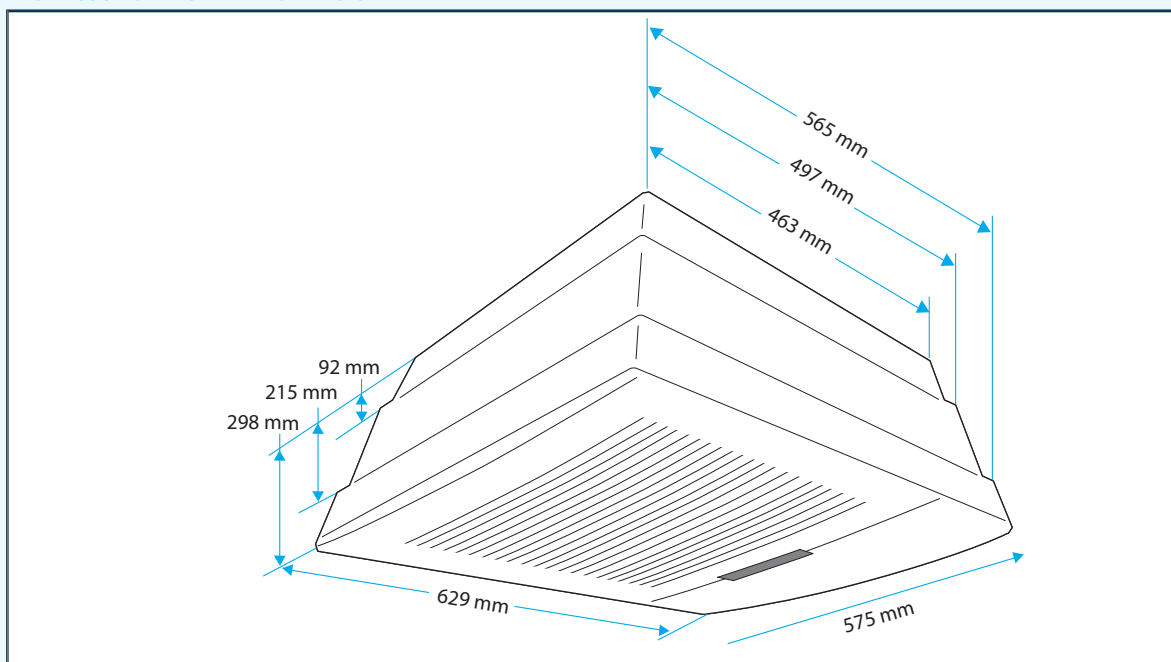
ABMESSUNGEN LUFTREINIGER VISIONAIR 2
