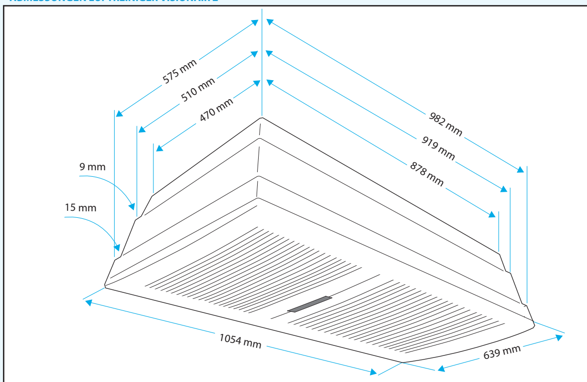
ABMESSUNGEN LUFTREINIGER VISIONAIR 2
